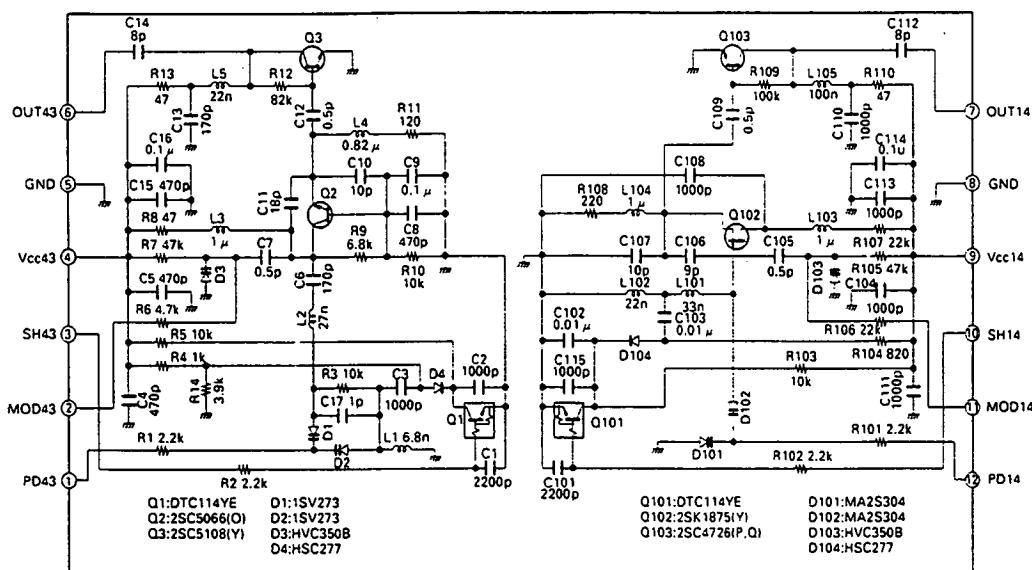
Fig.6 VCO circuit (KCH36)
